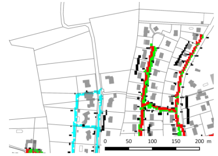
Réseau d'assainissement
