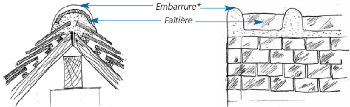
A - Le faîtage à tuiles faîtières et embarrures*.
