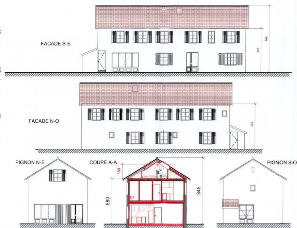
Elévations – état projeté, juillet 2021
