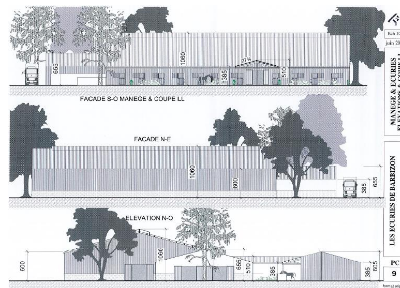
Elévation, coupe longitudinale
