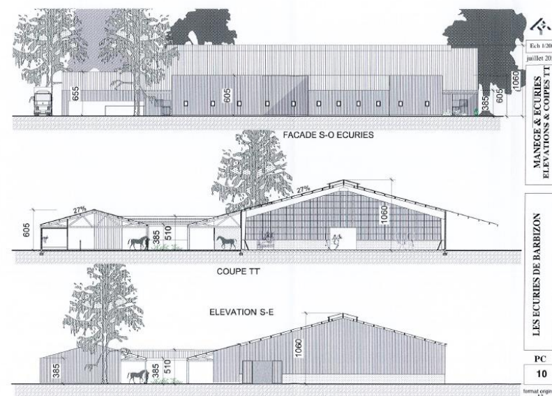
Elévation, coupe transversale
